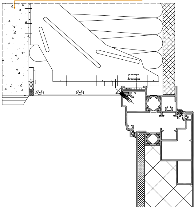
Base 52 : pose en neuf avec doublage
