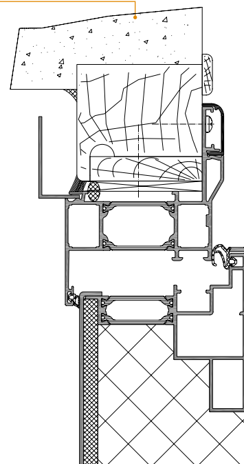
Base 72 : Rénovation pose frontale
